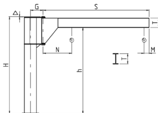
Gru a colonna Rotazione 290°
